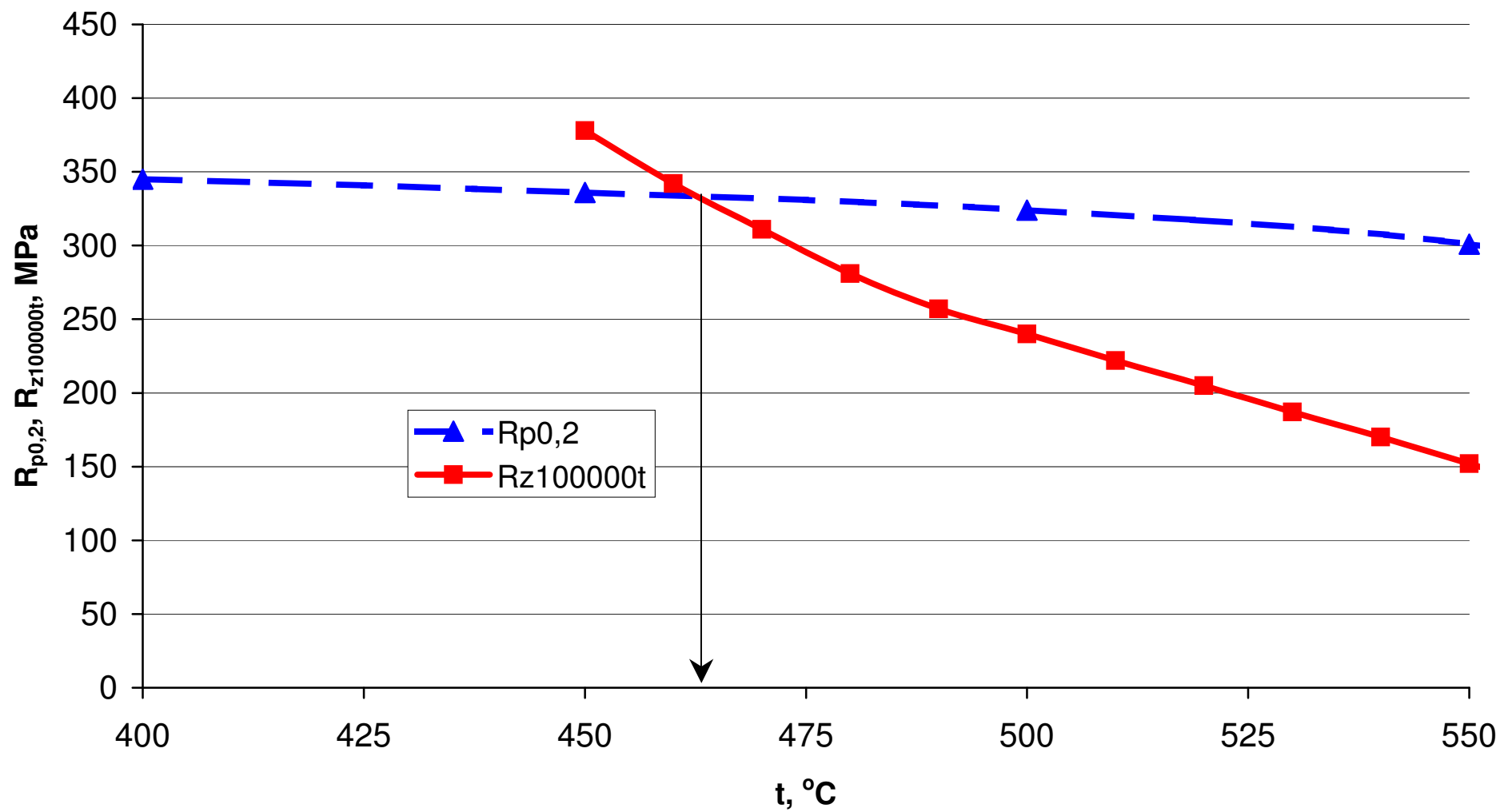
Temperatura graniczna dla stali 7CrMoVTiB10-10 (1.7378)
