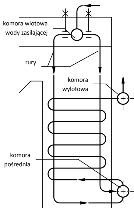
Rys. 21. Schemat zawieszenia podgrzewacza wody na rurach wieszakowych.
