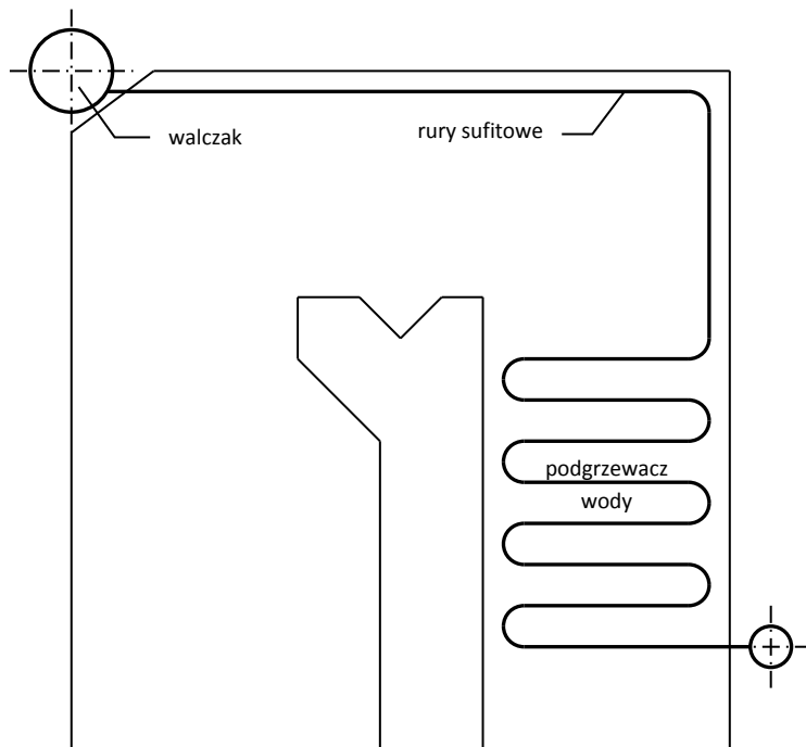
Rys. 22. Schemat połączenia podgrzewacza wody z walczakiem za pomocą rur sufitowych.
